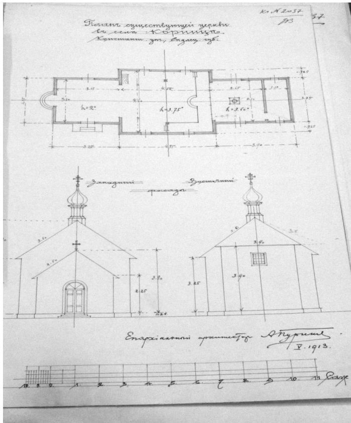
Il. 13. Schemat cerkwi w Kornicy, APL, Konsystorz Prawosławny w Chełmie, sygn. 2796, s. 25.
