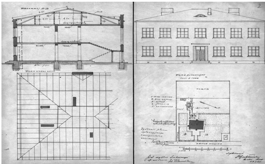
Il. 4. APL, Urząd Wojewódzki Lubelski, sygn. 2217, s. 2, Projekt 6-klasowej szkoły powszechnej w Kornicy z 1936 r.
