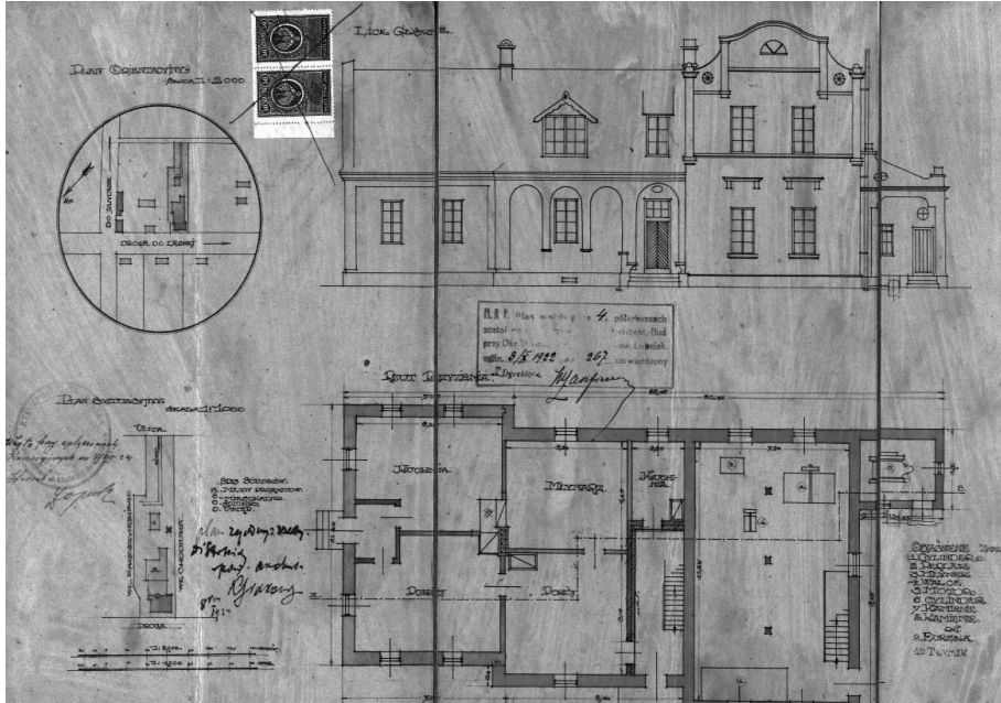
Il. 3. APL, Urząd Wojewódzki Lubelski, sygn. 1107, s. 2, Projekt młyna motorowego w Kornicy, 1922 r.
